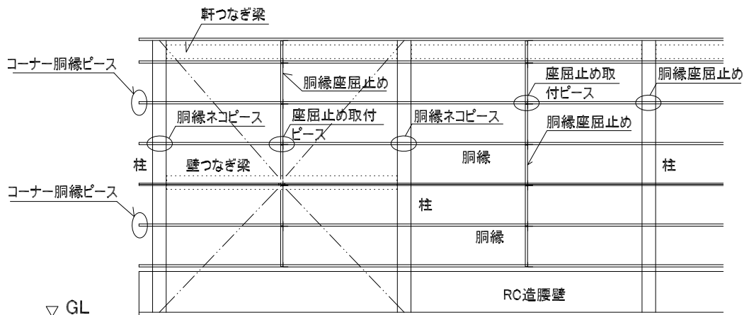
軸組図
