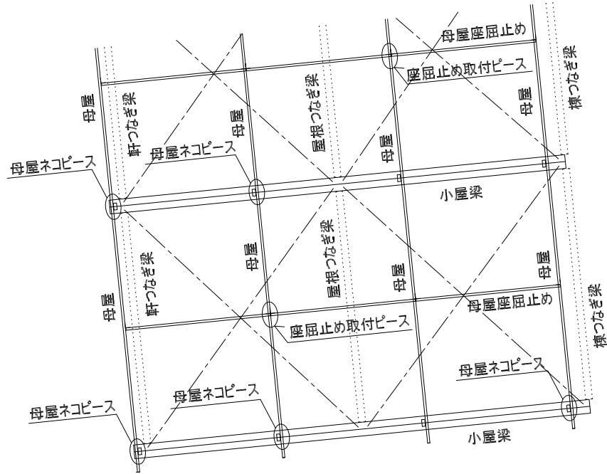
梁伏図
